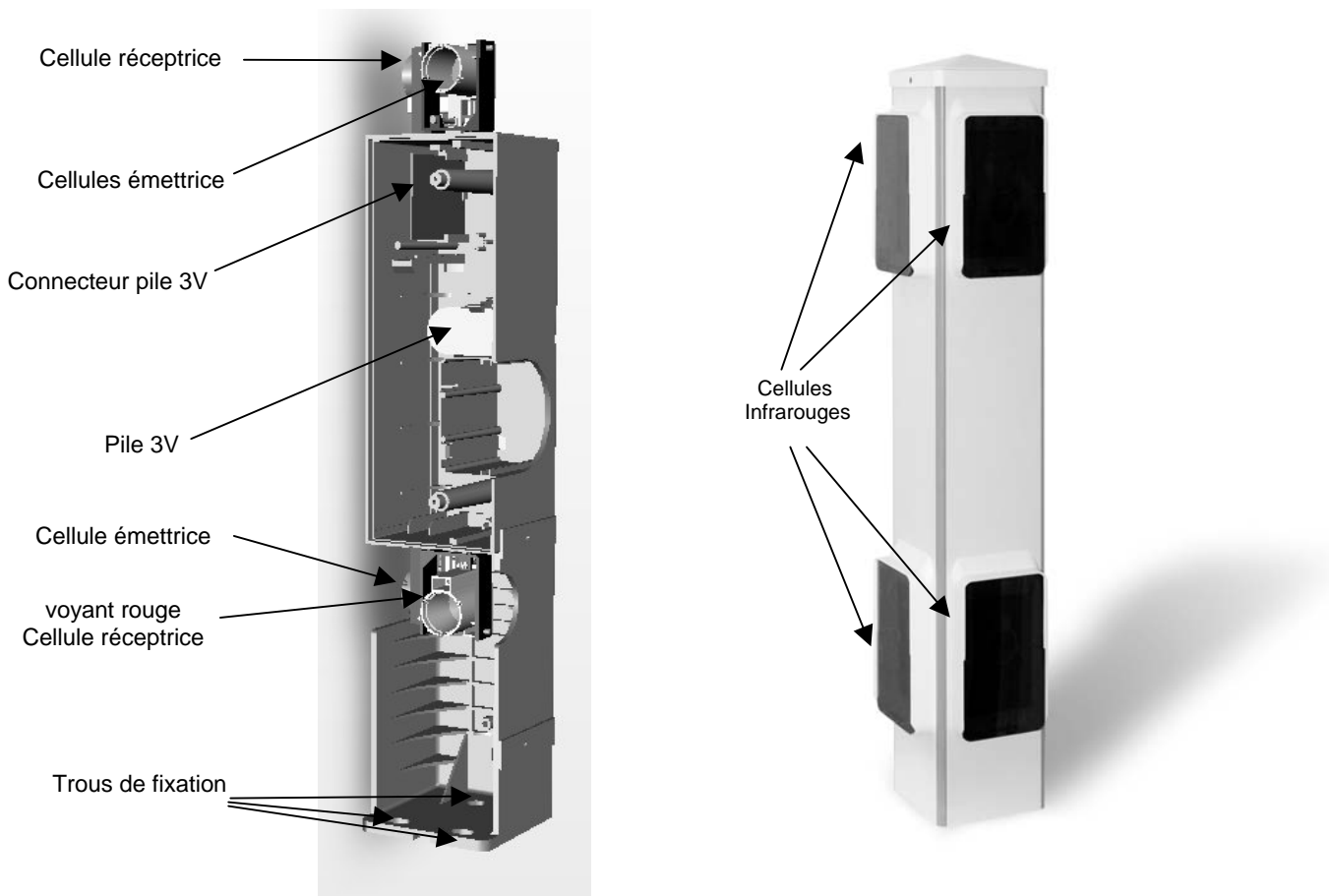
Figure 4 : borne esclave
